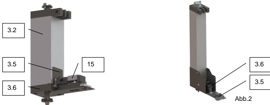
Поворотная опора для SRA 100, SRA 105
