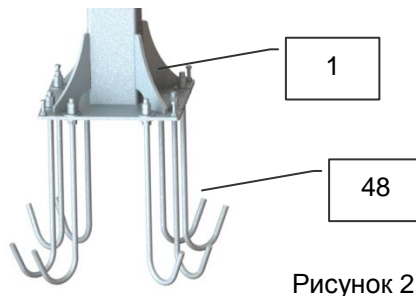
Анкерные болты
