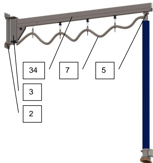
2.1.4 Настенный консольный поворотный кран с плоской стрелой
