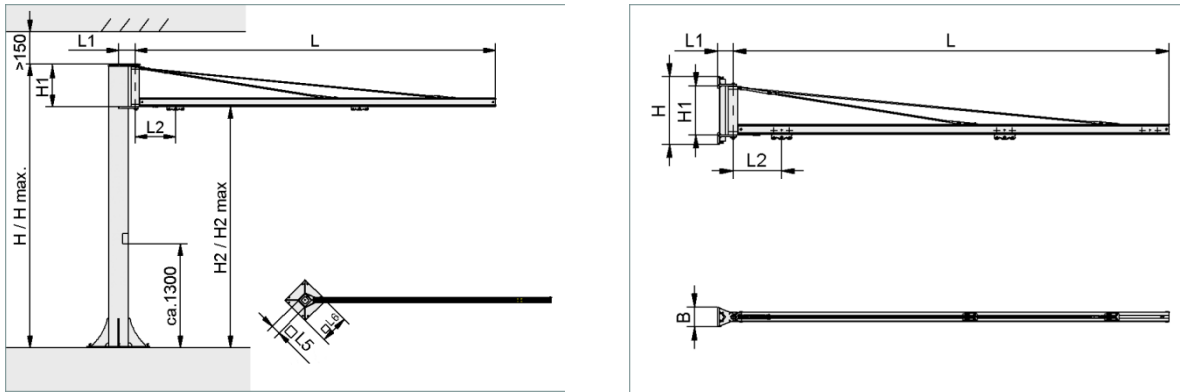
Консольный поворотный кран на колонне SK
